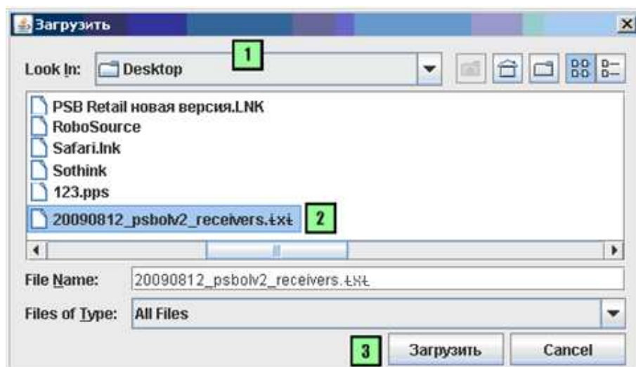
Рис. 23 Окно «Загрузить»
