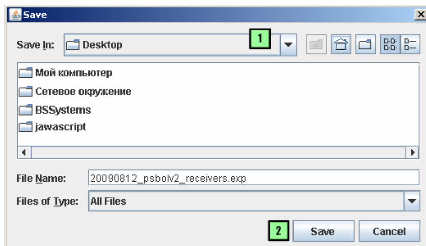
Рис. 20 Окно «Save»
